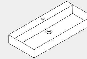
102x45xH12,5 cm ELLP102450QM
